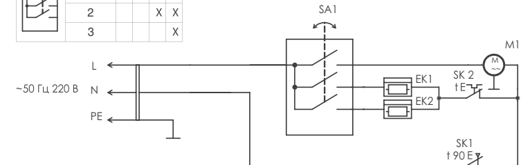
Схема электрическая тепловентилятора ЗТПЭ-5000_Ф_M2
