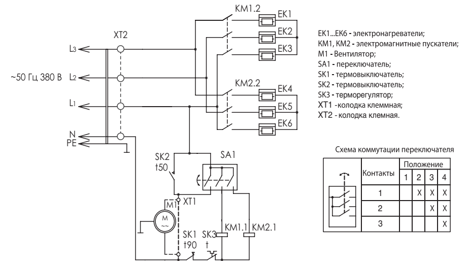
Схема электрическая тепловентиляторов ЗТПЭ-24000_Ф_M2
